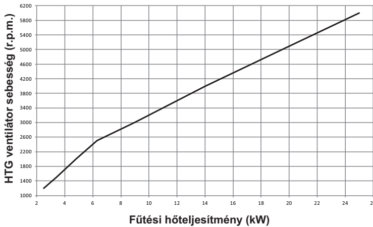
Hőteljesítmény görbe – ventilátor rpm (Qnrisc)
