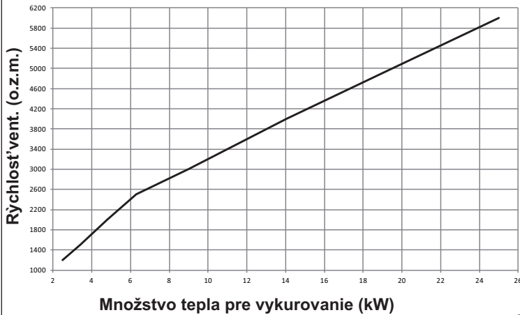
Krivka pre množstvo tepla – otáčky ventilátora (Qnrisc)
